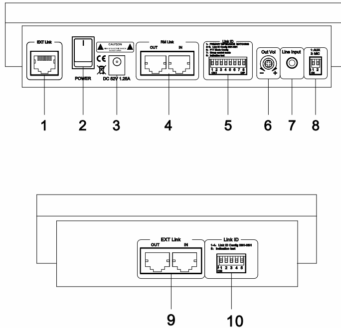
PAVA9008E Expansion Keyboard
